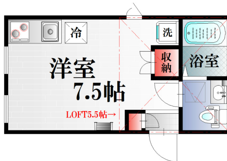
【間取り図】
